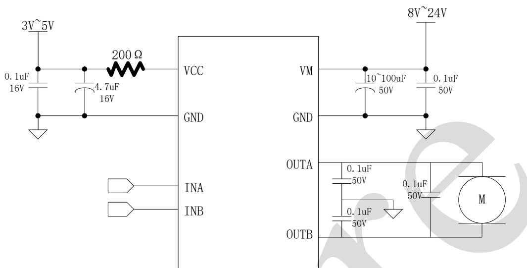
图 4、典型应用图
