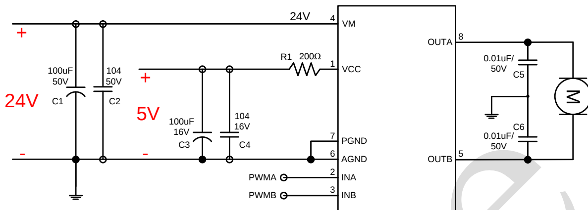
图 6、驱动风扇摇头电机应用线路图
