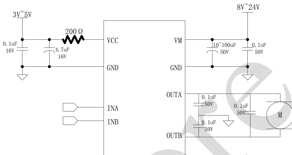
图 4、典型应用图
