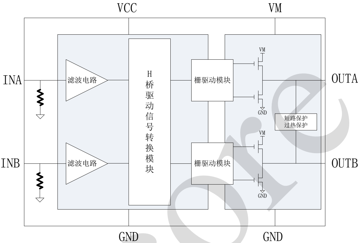
图 1、功能框图
