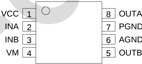
图 2、引脚图
