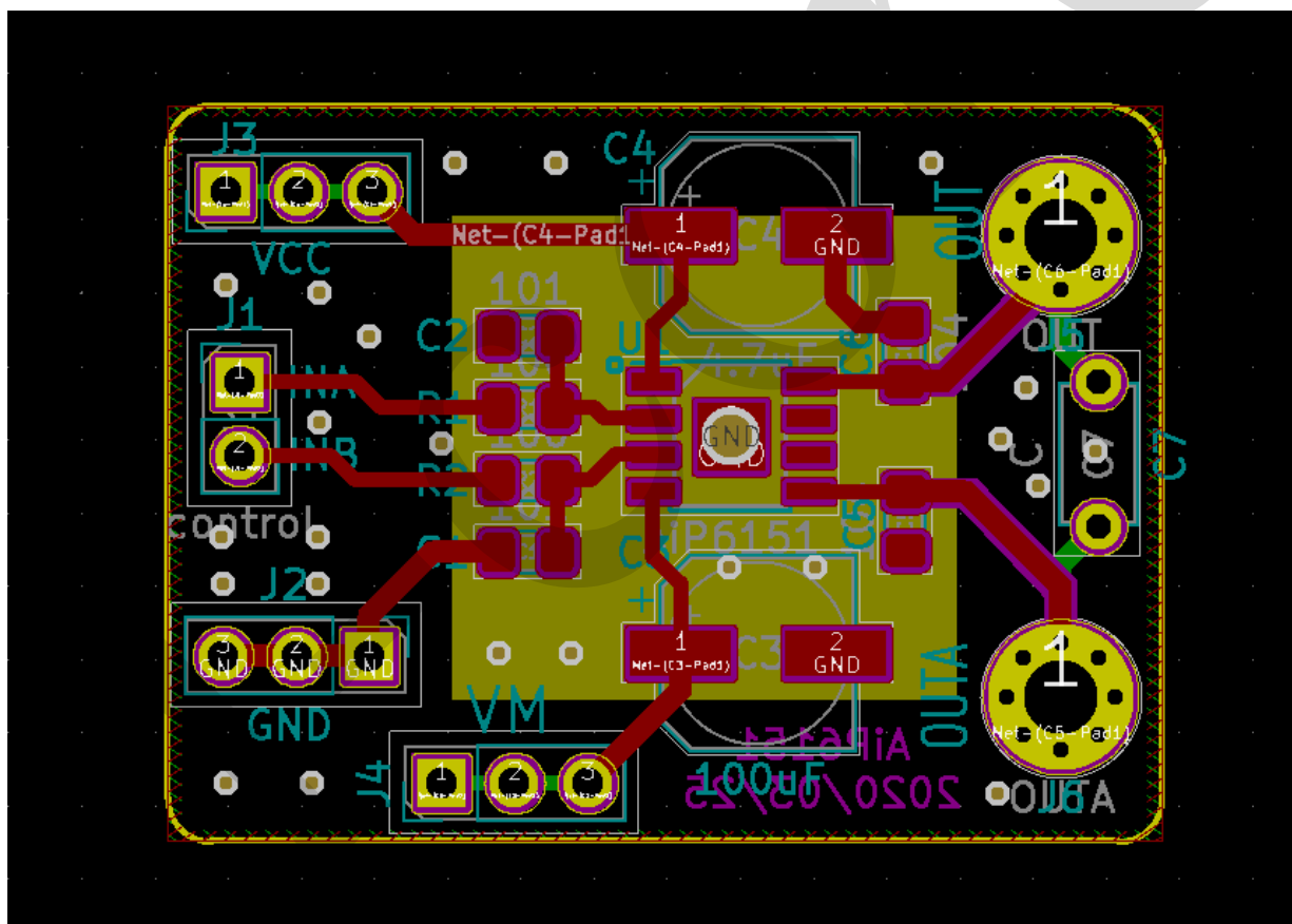
图 7、驱动风扇摇头电机 PCB 布版图
