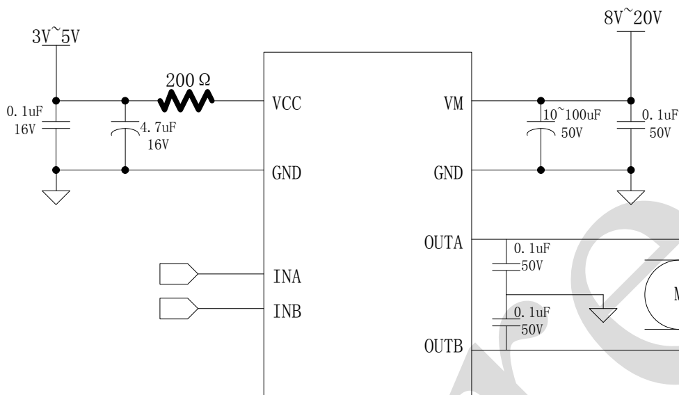
图 4、典型应用图
