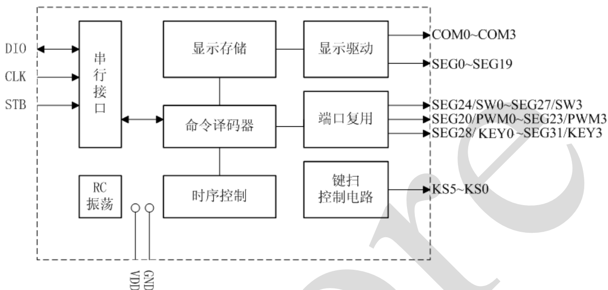
图 1、功能框图
