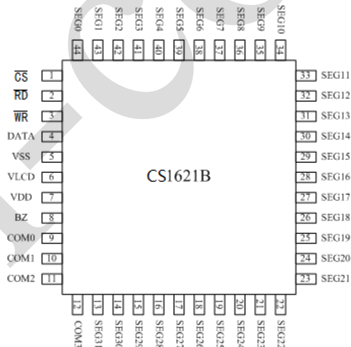
LQFP44 引脚图
