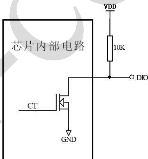
图 3、DIO 端口内部结构
