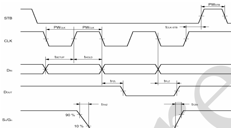
图 4、时序图
