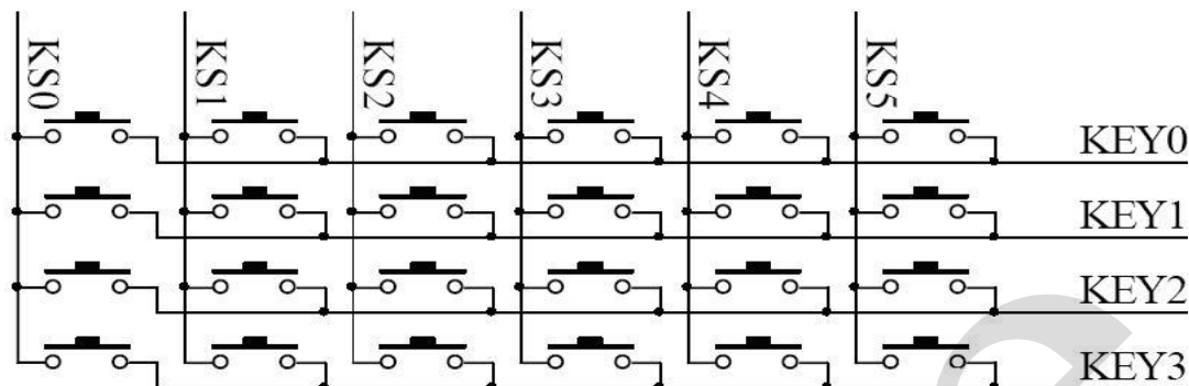
图 5、6×4bit 的键扫矩阵
