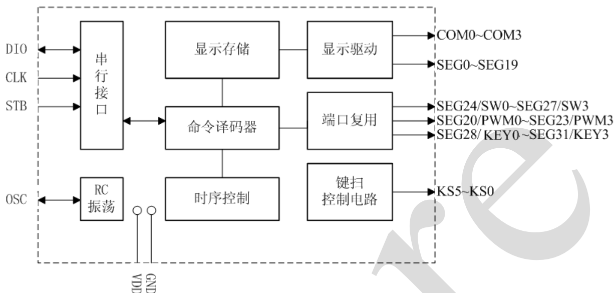
图 1、功能框图
