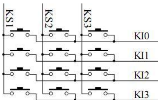
图 5、3×4bit 的键扫描矩阵
