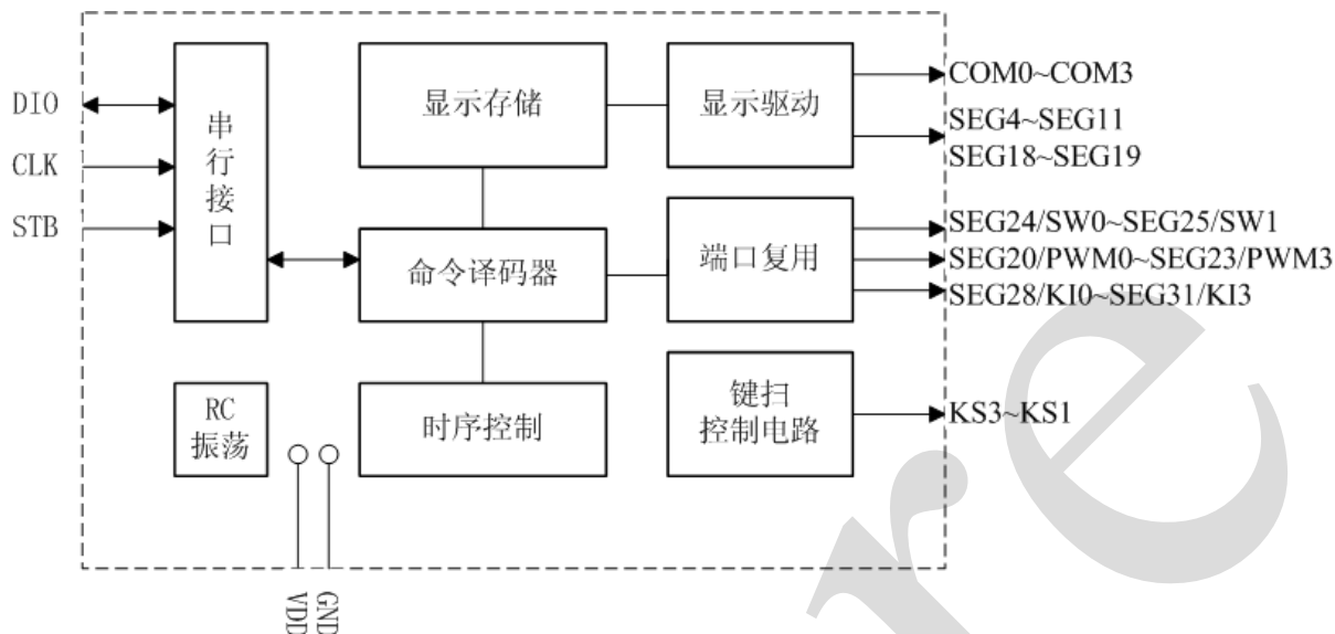
图 1、功能框图
