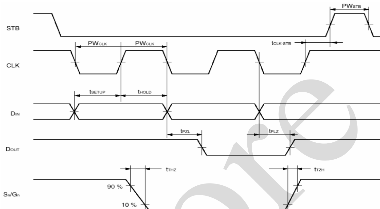
图 4、时序图
