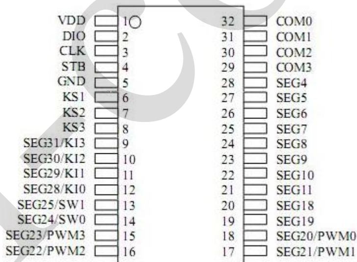
图 2、引脚排列图
