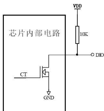
图 3、DIO 端口内部结构
