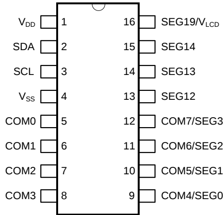
SOP16
