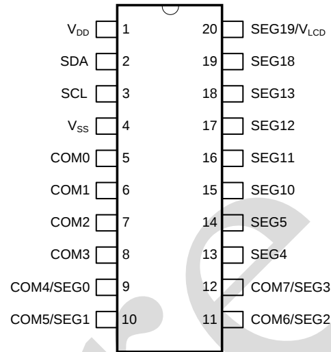
SOP20/SSOP20
