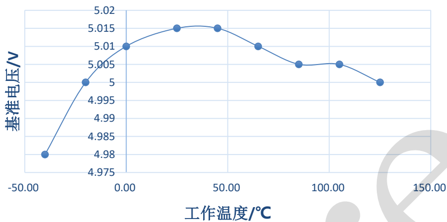
VREF温漂
