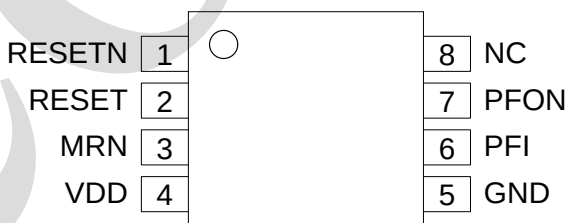
图 2-2、MSOP8 引脚图
