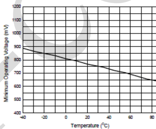
图8: 最小工作电压和温度的关系
