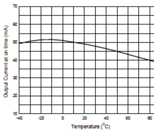
图9: 输出工作电流与温度的关系
