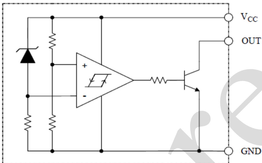
图 1: AiP7042 功能框图
