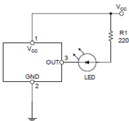
图13: 低电压指示器
