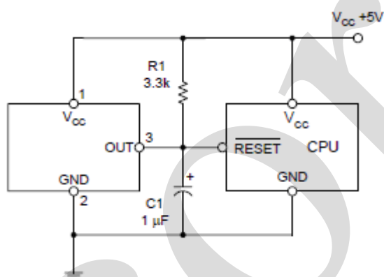
图14: CPU复位电路
