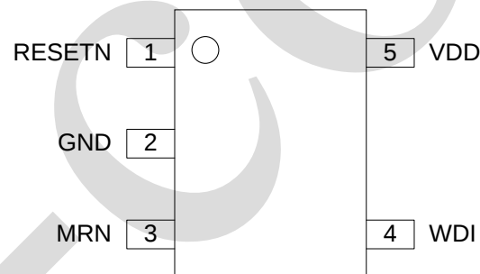
图 2、引脚图
