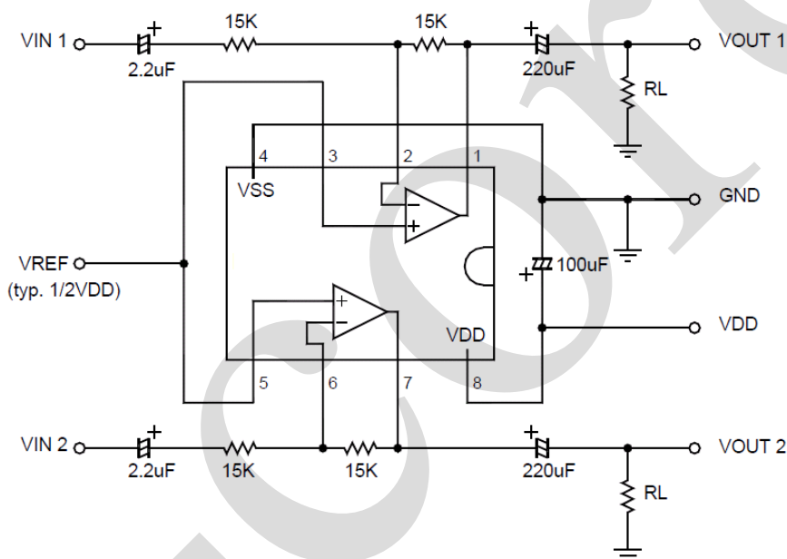
图 6、典型应用图
