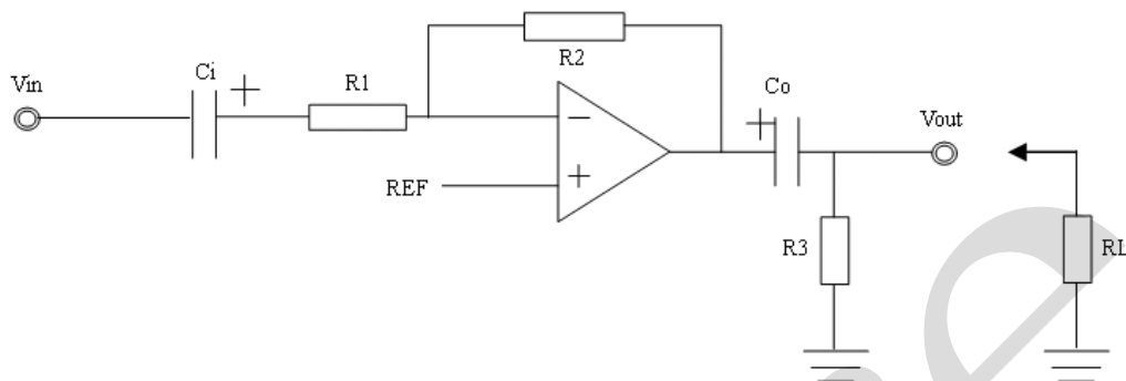
图 3、GW2308 典型应用图 (单个运算放大器)
