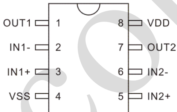
图 2、管脚排列图
