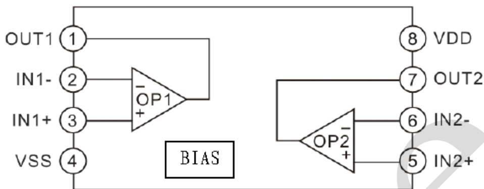
图 1、功能框图
