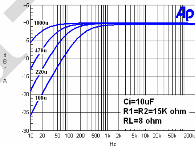
图 5、输出频率相应图
