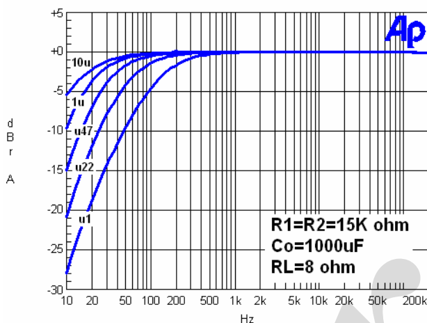
图 4、输入频率响应图
