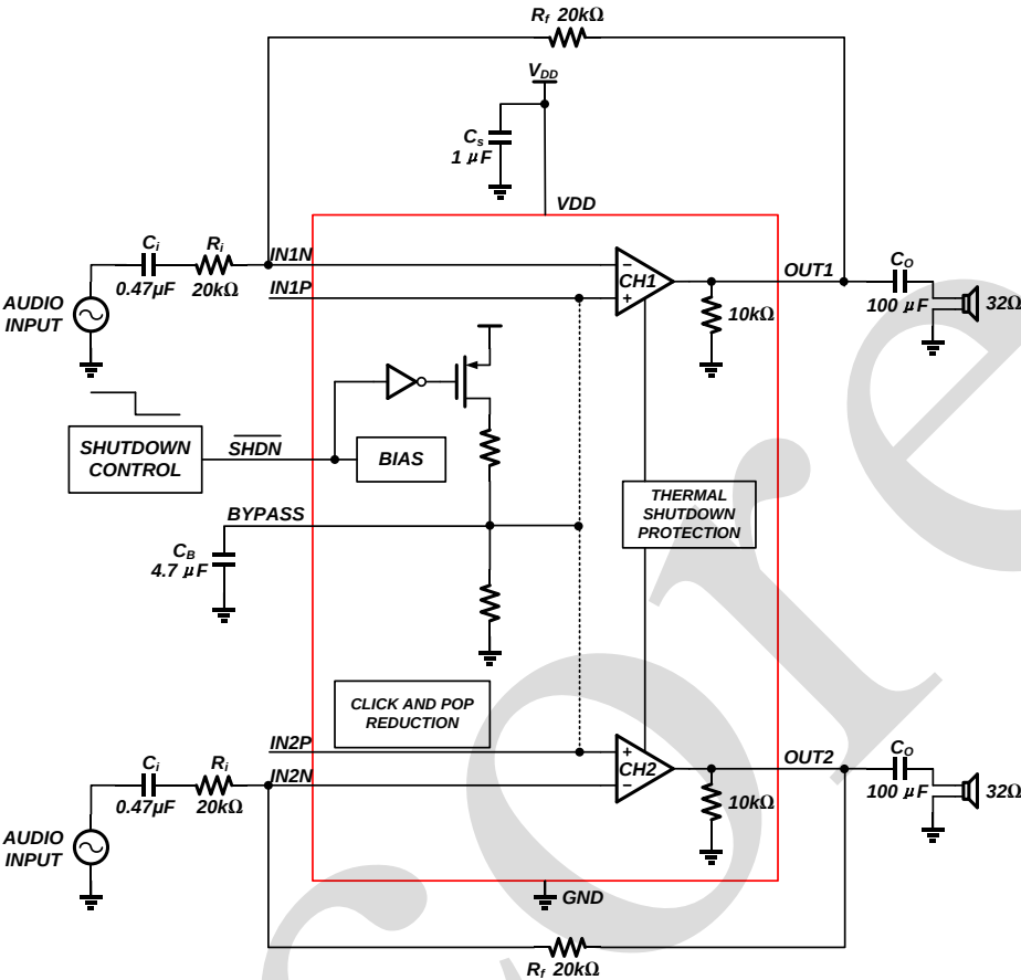
图 1、功能框图
