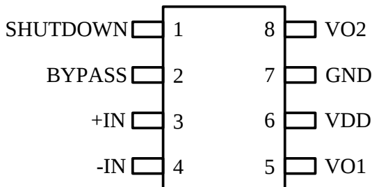
图 1、引脚排列
