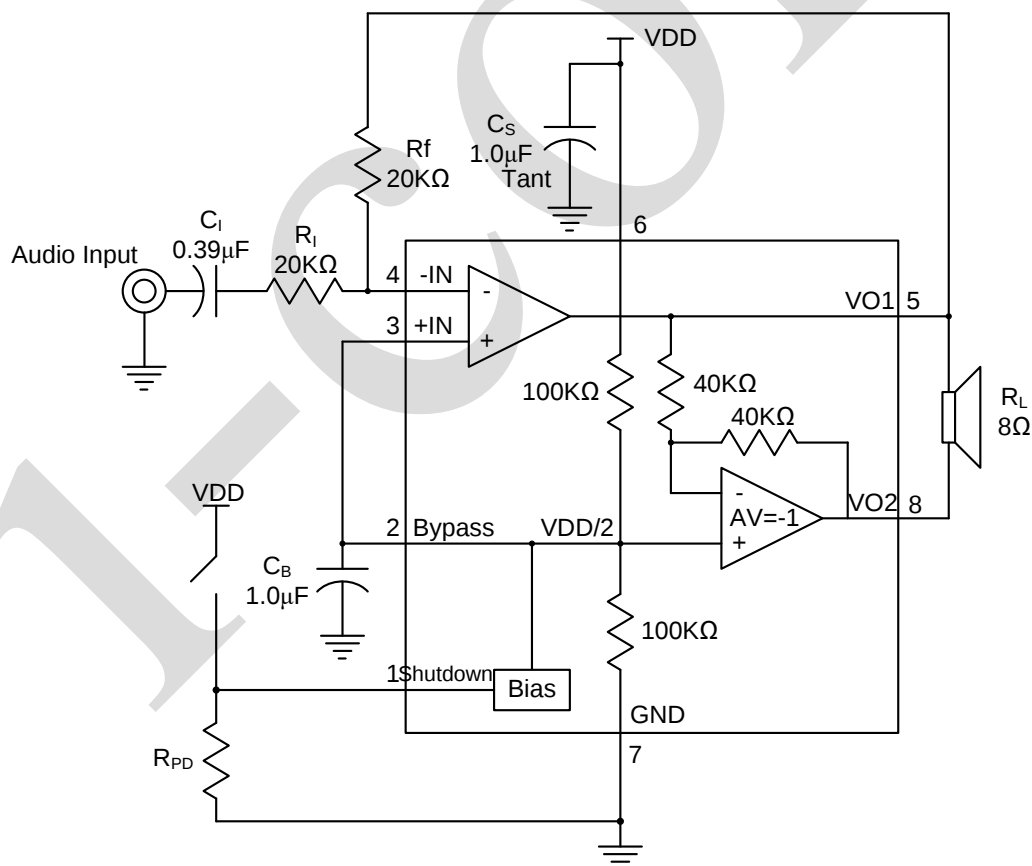
图 2、AiP4890 典型应用图
