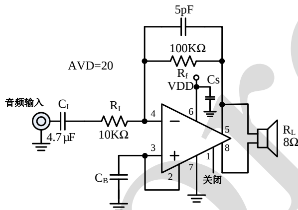
图3、高增益电路
