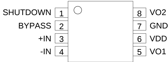
图 1、引脚排列
