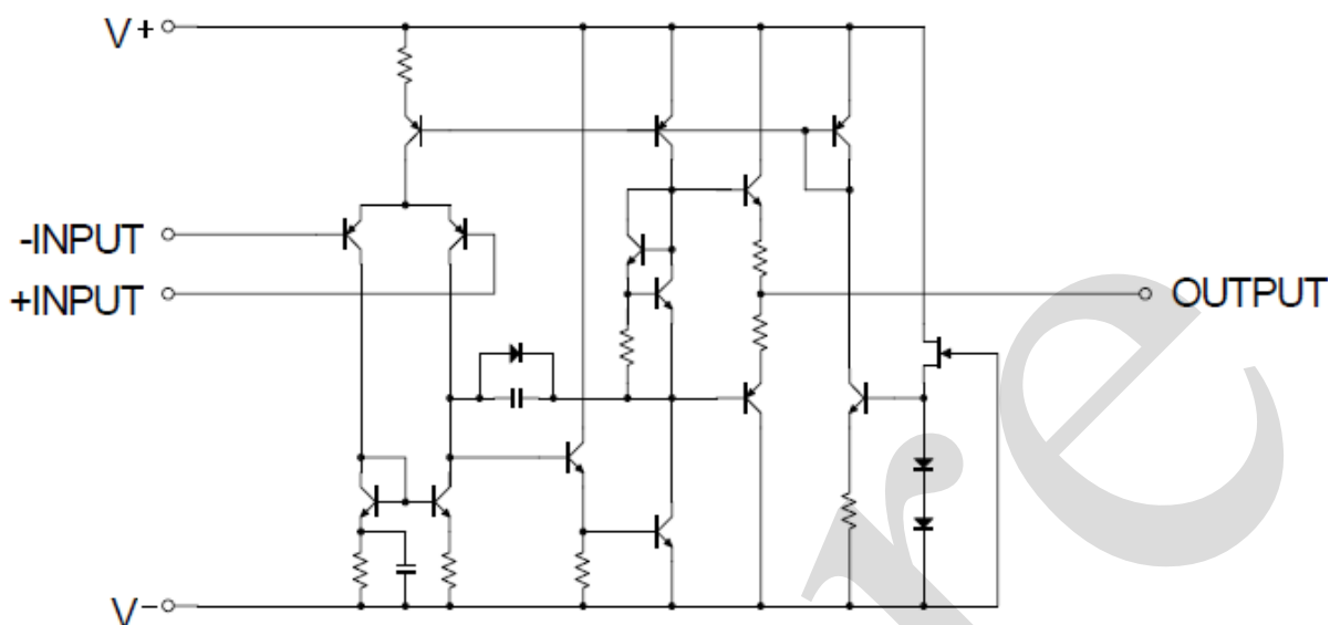
图 1 功能框图
