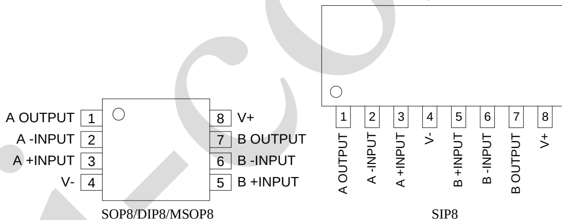
图 2 引脚图
