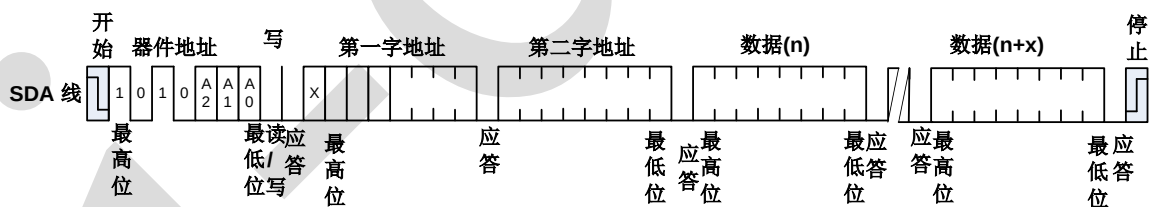
图 9、页写
