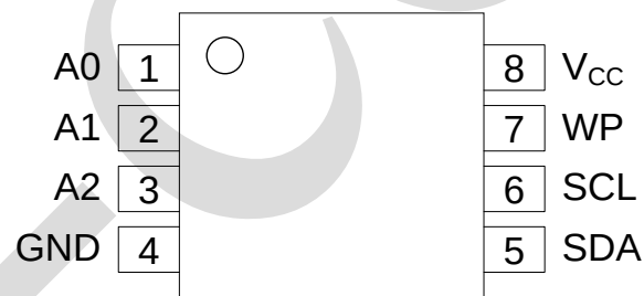
图 2、引脚排列图
