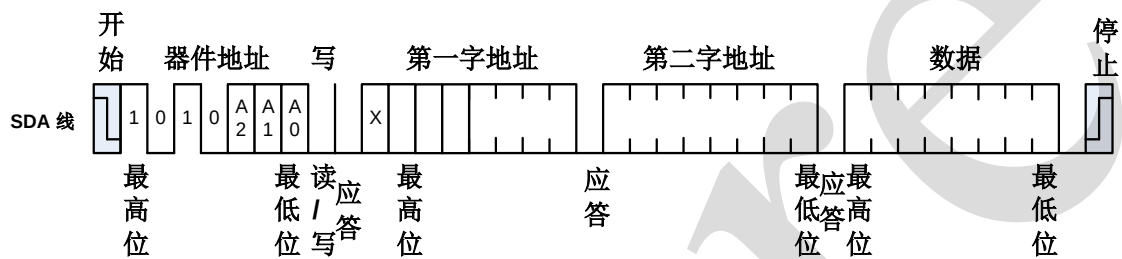
图 8、字节写
