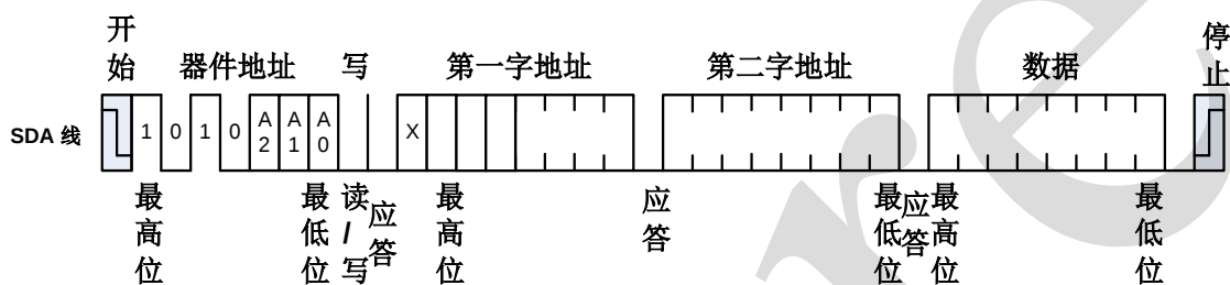
图 8、字节写
