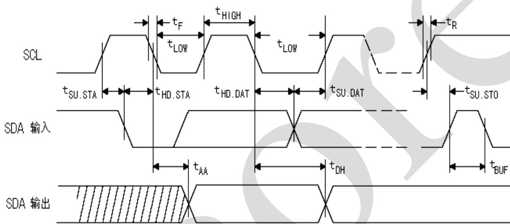
图 5、总线时序
