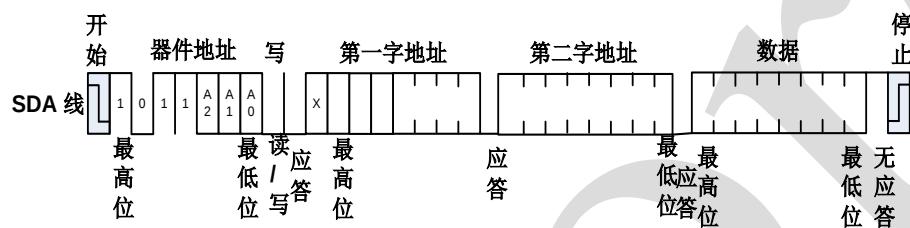
图 13、读锁存状态
