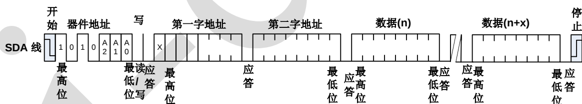
图 9、页写
