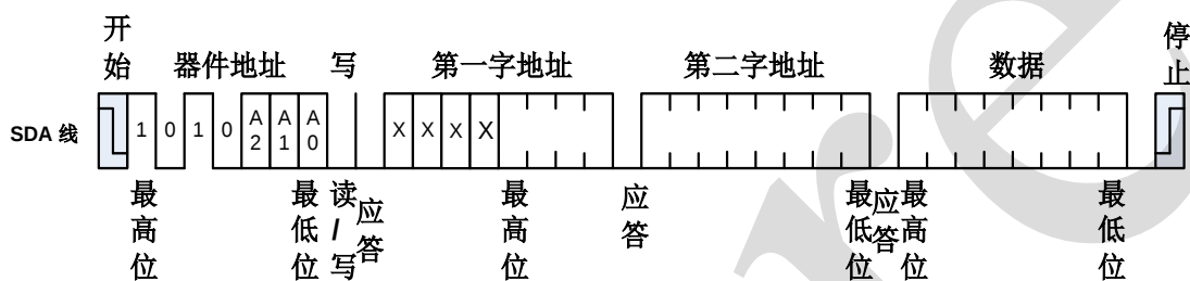
图 8、字节写
