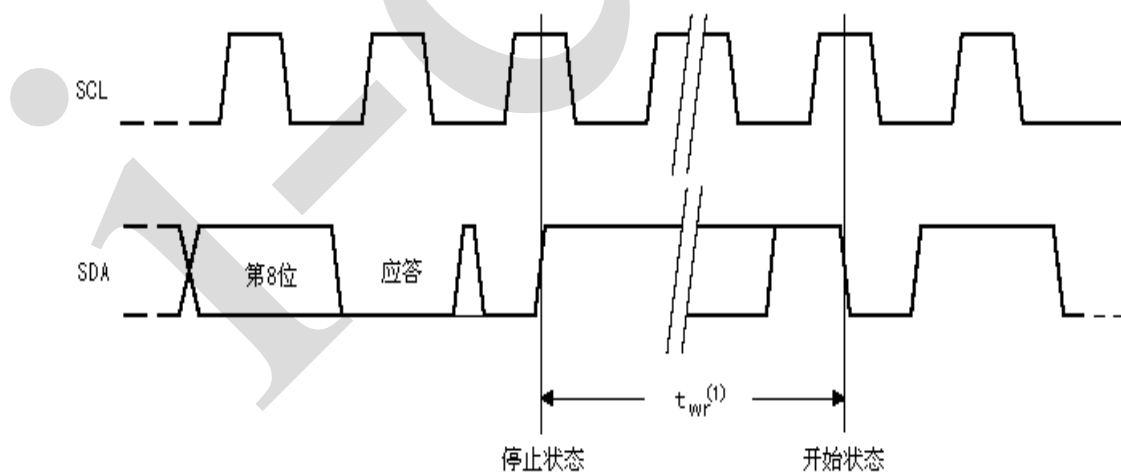
图 6、写周期时序
