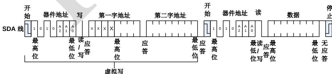
图 11、随机地址读操作
