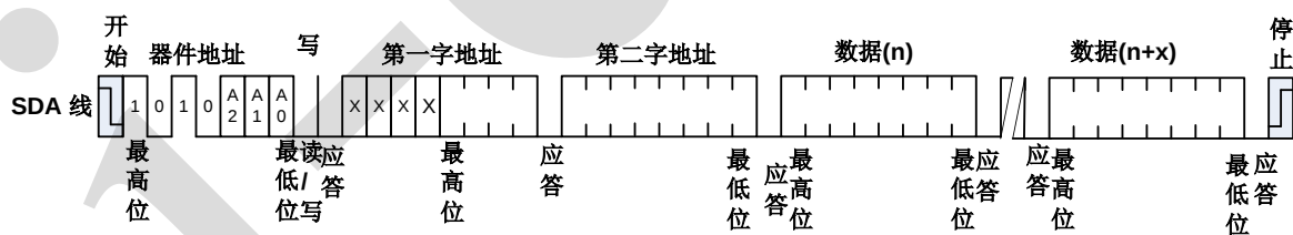
图 9、页写
