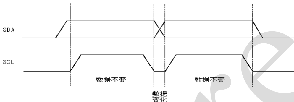
图 3、数据有效时序图
