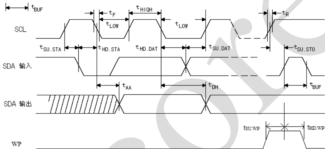
图 5、总线时序
