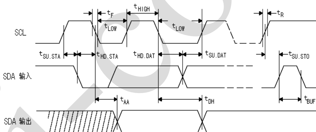
图 5、总线时序
