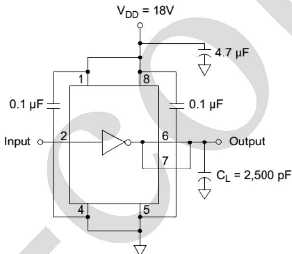
图 3 测试线路图
