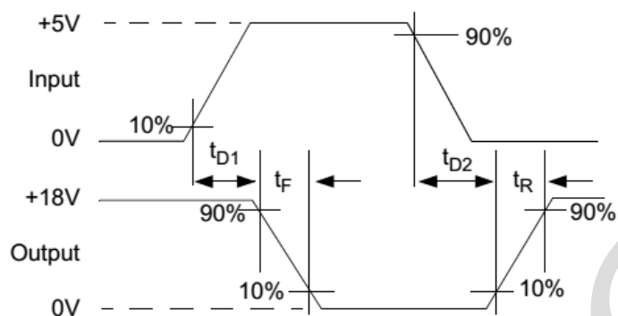
图 2 输入到输出的传输延时
