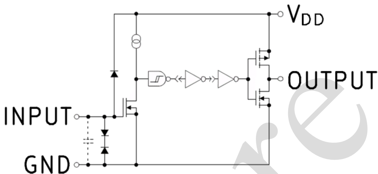
图 1 功能框图
