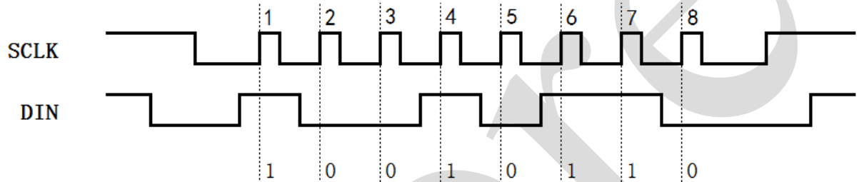
图 2 单字节通信
