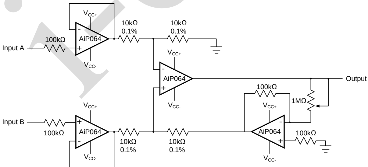
仪表放大器
