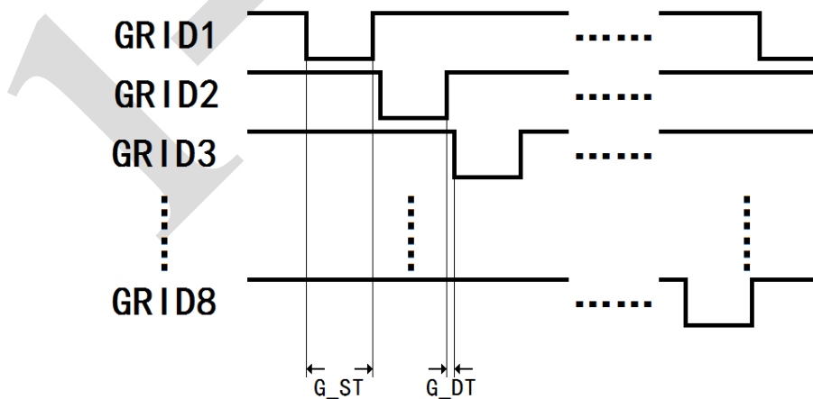
图 5 GRID 扫描波形示意图
