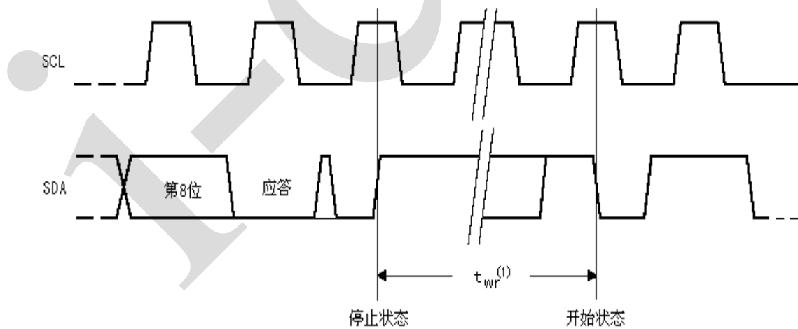
图 6、写周期时序
