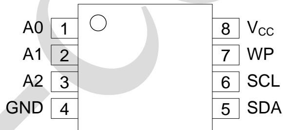
图 2、引脚排列图
