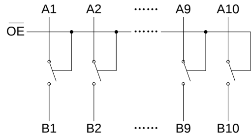
图 1 逻辑框图
