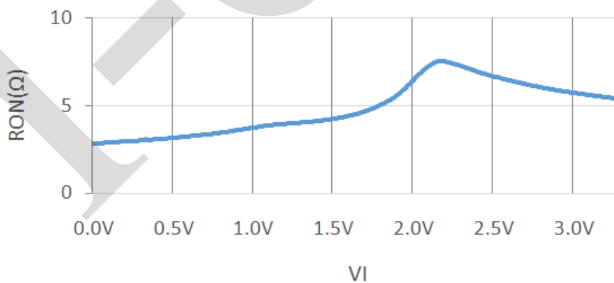
图 6 导通电阻与输入电压的关系 ( V_{CC}=3.3V , I_{SW}=24mA , T_{amb}=25^{\circ}C )
