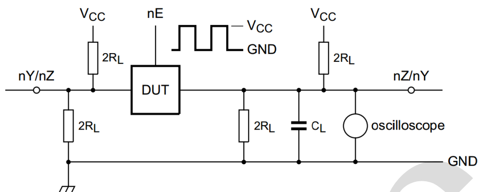
a. Circuit
