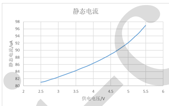
图 1 静态电流与供电电压
