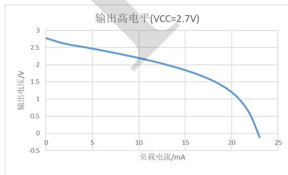
图 3 输出高电平与负载电流 ( V_{\text{CC}}=2.7\text{V} )
