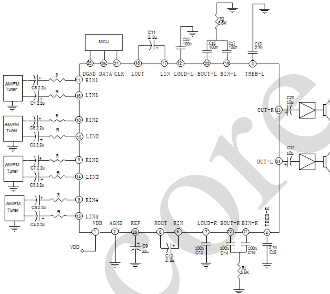
图 3、典型应用图
