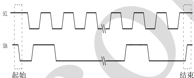
图 5、数据传输
