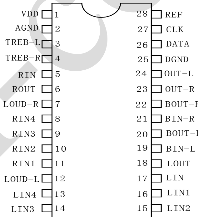
图 2、引脚排列
