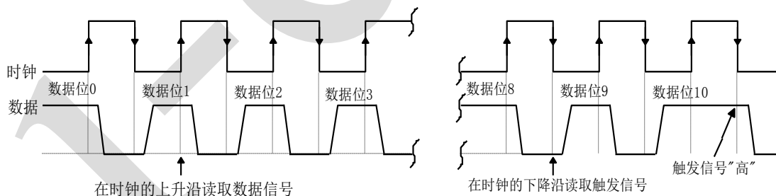
图 5、时序图
