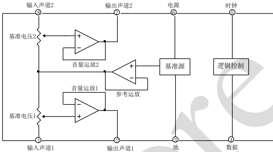
图 1、功能框图
