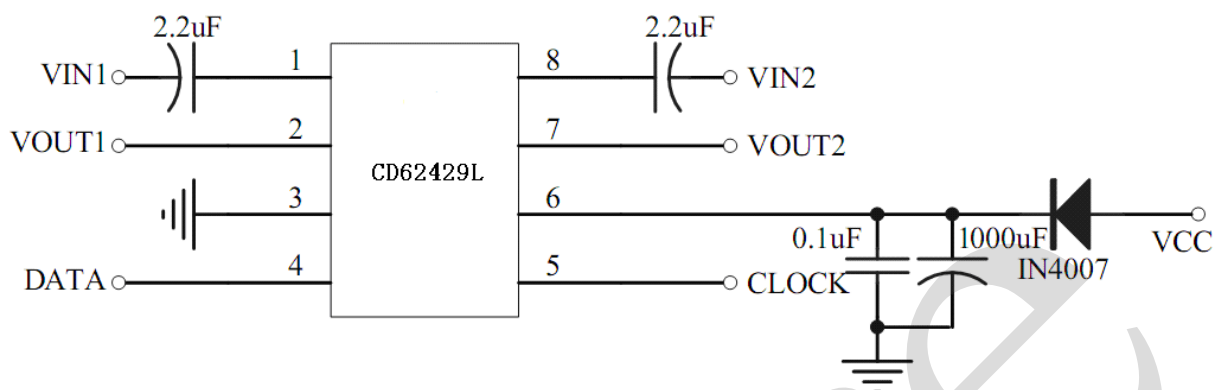
图 4、应用线路
