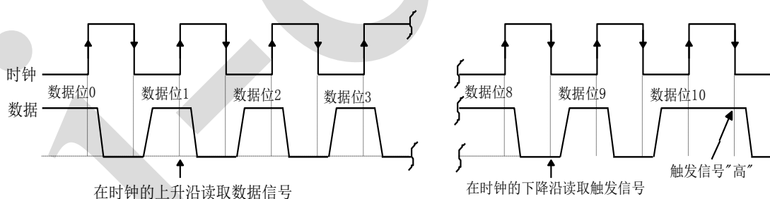
图 5、时序图
