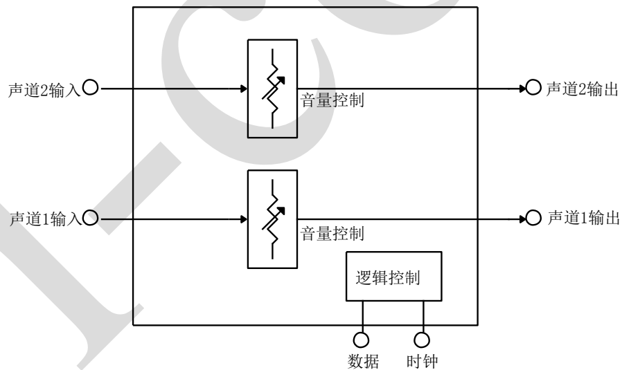
图 2、系统配置
