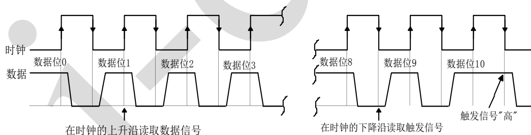
图 5、时序图
