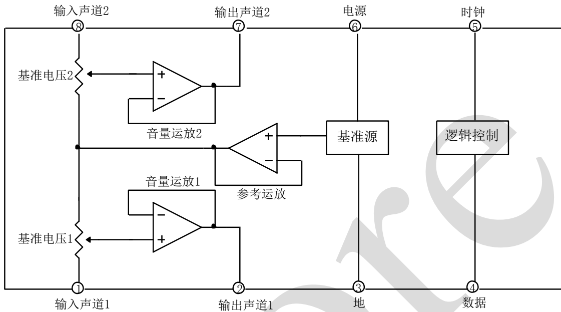
图 1、功能框图
